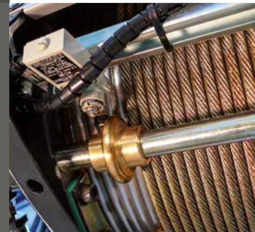
Rope guide
